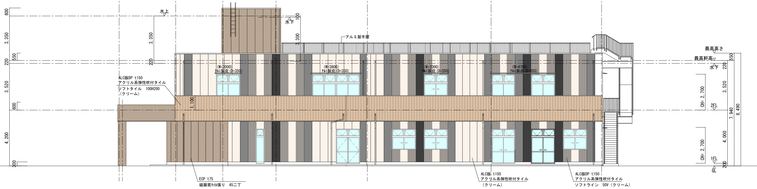
南側立面図 1/100
